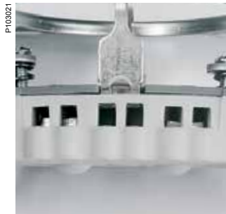
Kablo terminalleri hizalanmış olduğundan tüm kablolar tek seferde aynı uzunlukta kesilebilir. Çıkışlarda yarı açık terminaller bulunmaktadır.
